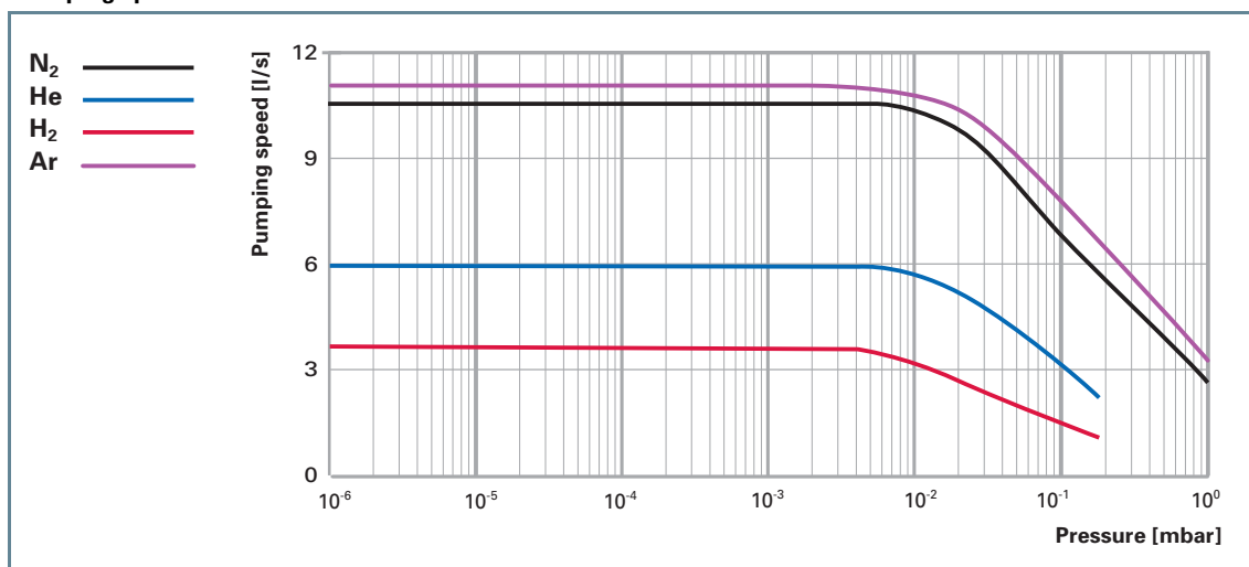
HiPace™ 10
